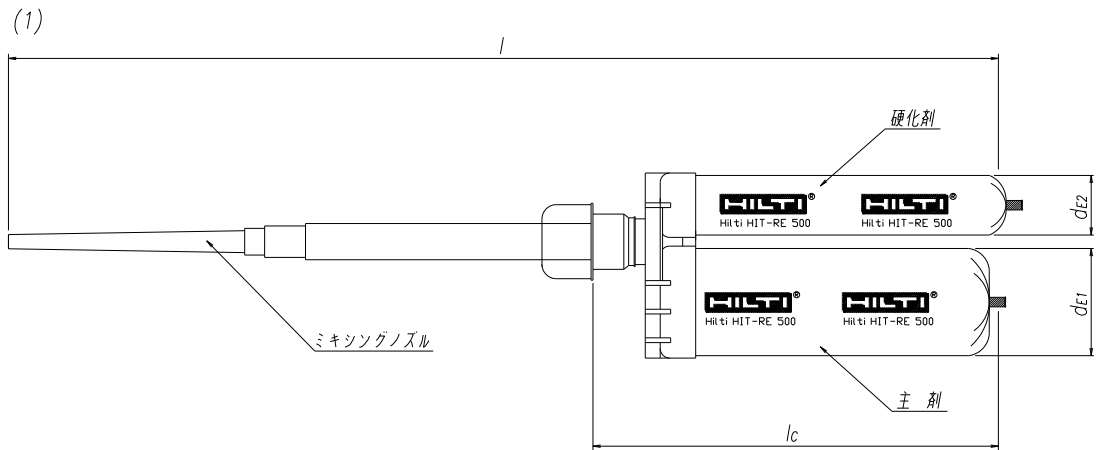
(1)本体・ミキシングノズル [単位:mm]
