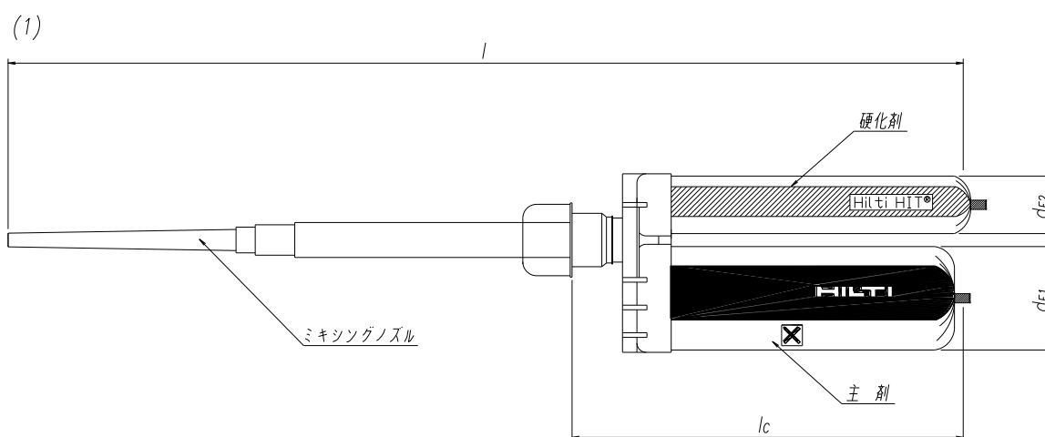
(1)本体・ミキシングノズル
