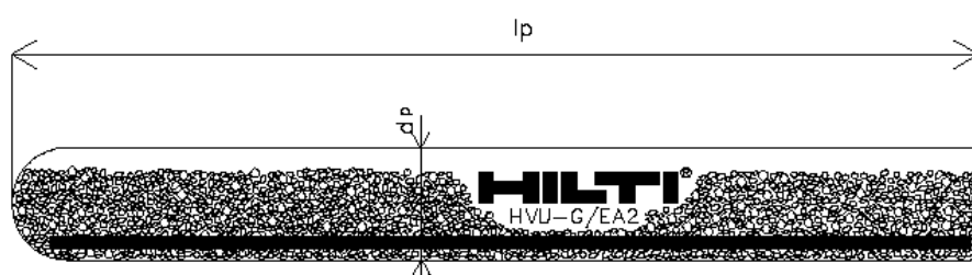
HVU-G/EA2 カプセル
