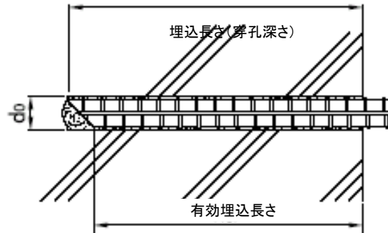
埋込長さ(穿孔深さ)と有効埋込長さ
